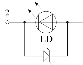
Zener Diode
